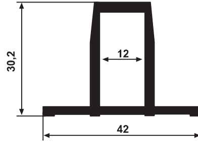
YG 2393 0,668 kg/m
