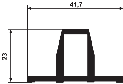
YG 1182 0,545 kg/m
