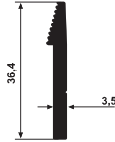
YG 3087 0,345 kg/m
