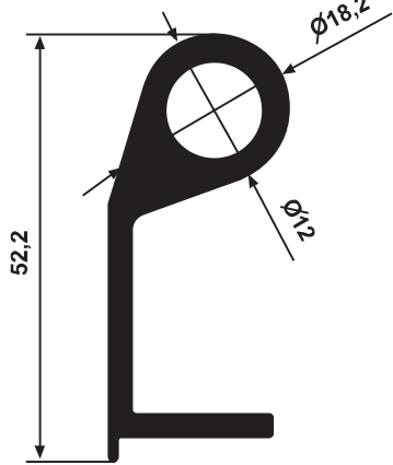
YG 2405 0,930 kg/m
