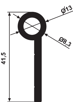
YG 2743 0,465 kg/m
