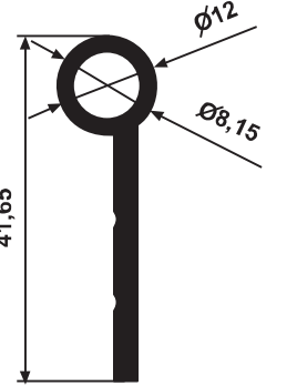
YG 3085 0,390 kg/m
