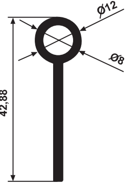
YG 2398 0,362 kg/m
