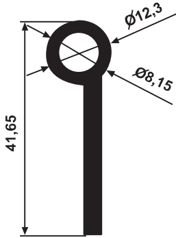
YG 2401 0,450 kg/m
