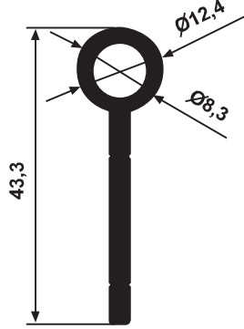
YG 2746 0,422 kg/m
