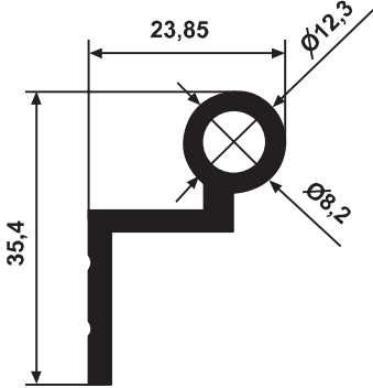
YG 2549 0,451 kg/m
