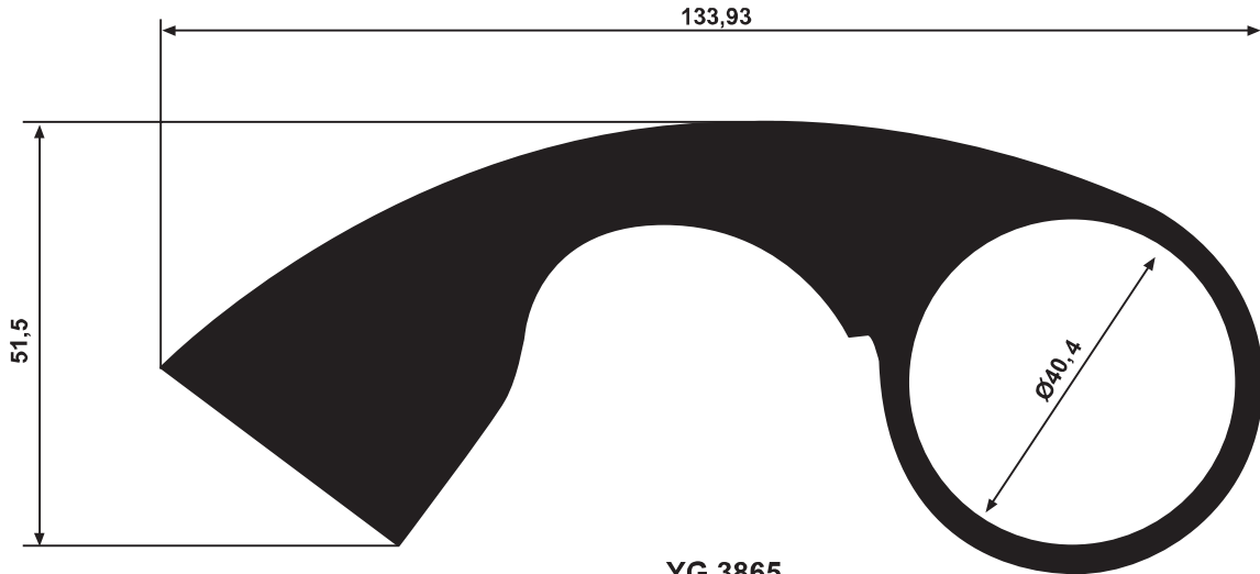
YG 3865 6,529 kg/m
