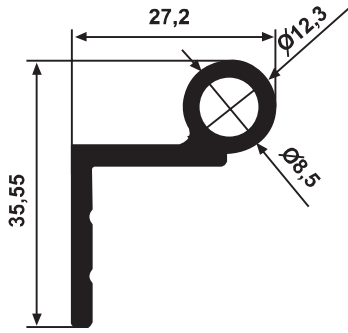
YG 3484 0,448 gr/m
