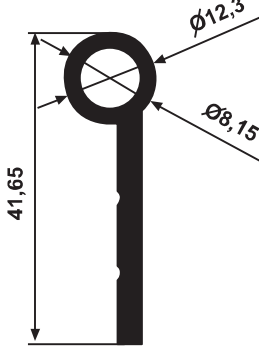
YG 1433 0,440 kg/m
