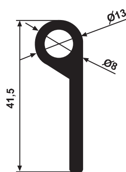
YG 3807 0,532 kg/m
