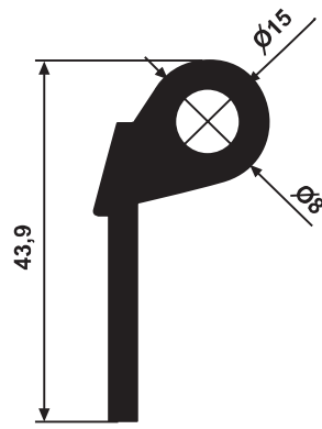
YG 2639 0,789 kg/m
