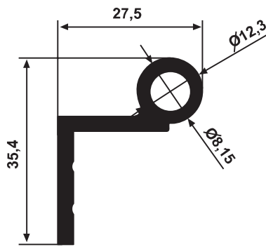
YG 1435 0,490 kg/m
