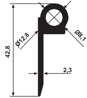
YG 2402 0,468 kg/m
