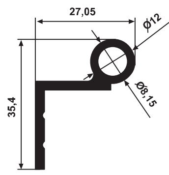
YG 3084 0,447 kg/m
