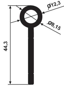
YG 2899 0,440 kg/m
