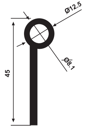
YG 4177 0,444 kg/m
