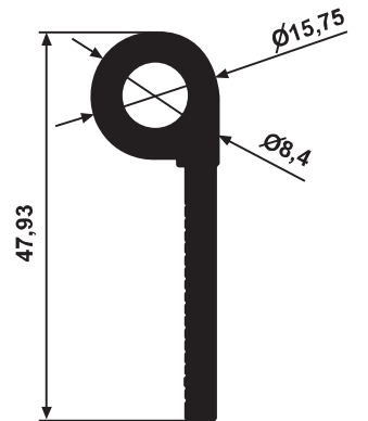
YG 3442 0,747 kg/m
