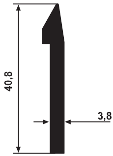
YG 2228 420 kg/m
