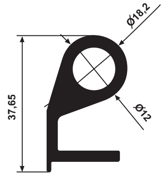
YG 2404 0,820 kg/m
