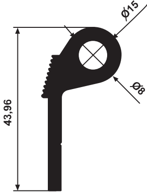
YG 3086 0,783 kg/m
