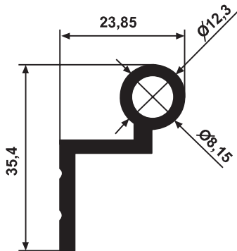
YG 1434 0,462 kg/m
