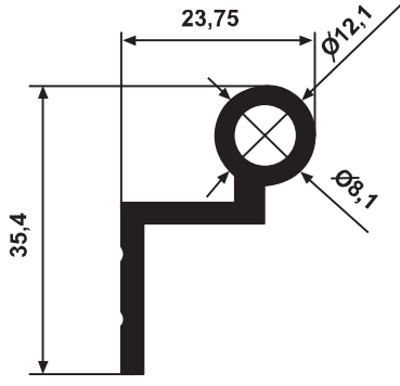
YG 3294 440,6 kg/m
