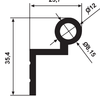
YG 3083 0,422 gr/m
