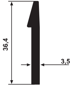
YG 2638 0,353 kg/m
