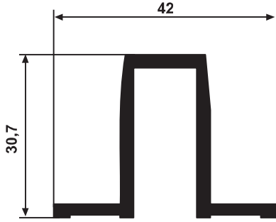
YG 1180 0,612 kg/m
