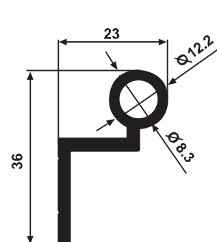
YM 2745 0,430 kg/m
