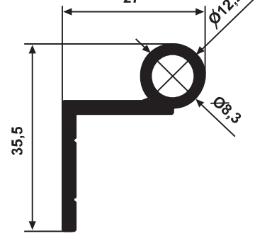
YG 2744 0,451 kg/m
