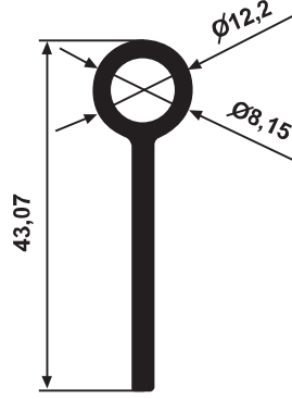
YG 2705 0,385 kg/m
