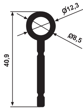
YG 3485 0,393 kg/m
