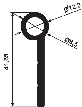
YG 3486 0,408 kg/m
