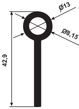
YG 2716 0,462 kg/m
