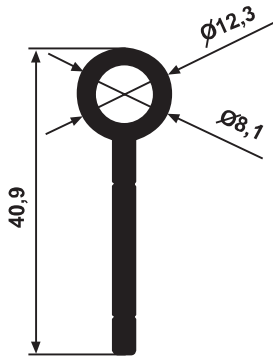
YG 2796 0,406 kg/m
