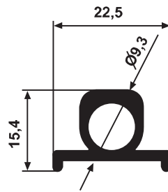
YG 2703 0,294 kg/m
