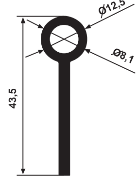
YG 3077 0,445 kg/m
