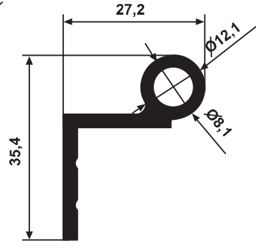
YG 3295 0,464 kg/m
