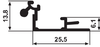
YG 3218 0,198 kg/m
