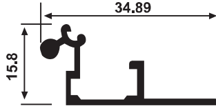
YG 2325 0.234 kg/m
