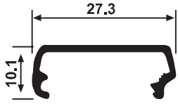
YG 2038 0,146 kg/m
