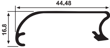
YG 2409 0,283 kg/m
