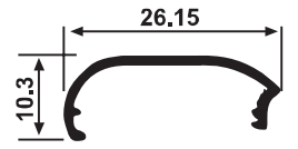
YG 2314 0,132 kg/m
