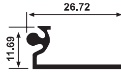
YG 2562 0,145 kg/m
