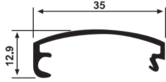
YG 1305 0,195 kg/m
