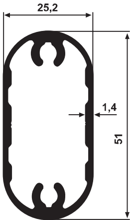
YG 4805 0,754 kg/m
