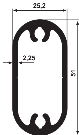
YG 4806 0,926 kg/m
