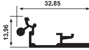
YG 1304 0,260 kg/m
