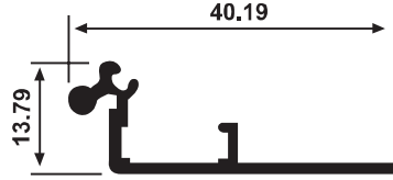
YG 2410 0,263 kg/m
