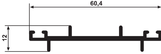
YG 3991 0,425 kg/m
