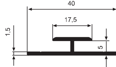
YG 3054 0,250 kg/m
