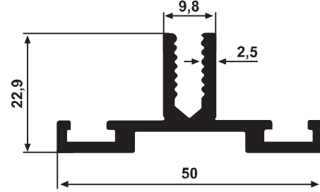
YG 4570 0,615 kg/m
