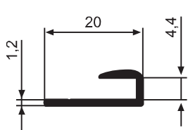
YG 1125 0,109 kg/m
