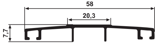
YG 5078 0,312 kg/m
