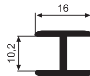
YG 1123 0,132 kg/m
