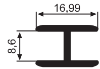
YG 1124 0,113 kg/m
