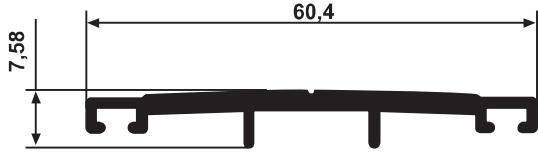
YG 3992 0,462 kg/m
