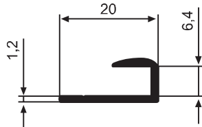
YG 1251 0,115 kg/m
