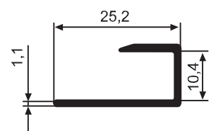
YG 1252 0,139 kg/m
