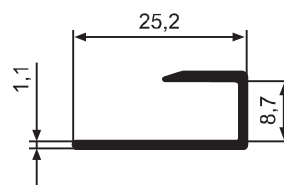
YG 1098 0,133 kg/m
