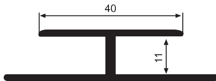
YG 3246 0,461 kg/m
