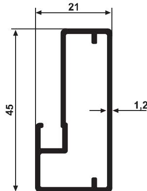
YG 3427 0,461 kg/m
