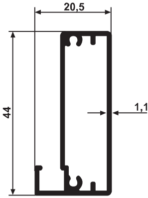
YG 3682 0,428 kg/m
