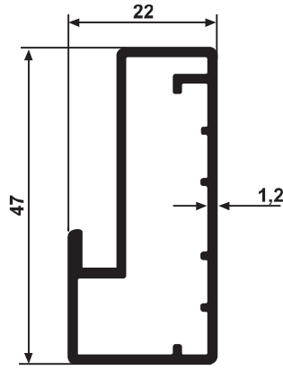
YG 2114 0,497 kg/m
