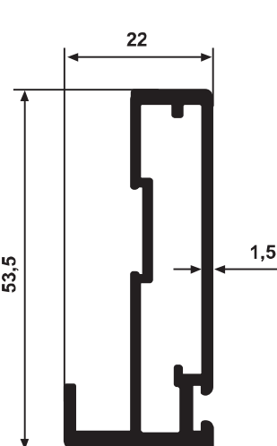
YG 2428 0,669 kg/m
