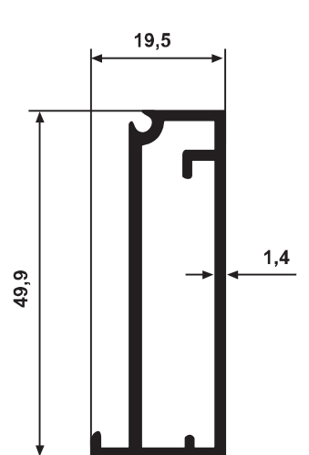
YG 4131 0,505 kg/m
