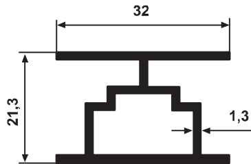
YG 2082 0,419 kg/m
