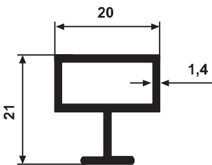
YG 2384 0,283 kg/m
