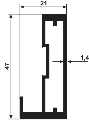
YG 2092 0,624 kg/m
