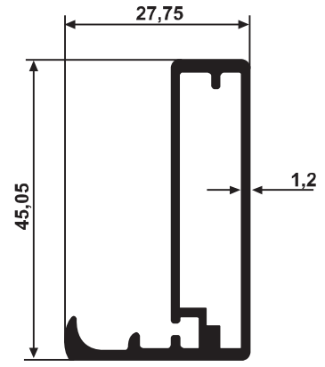
YG 3907 0,512 kg/m
