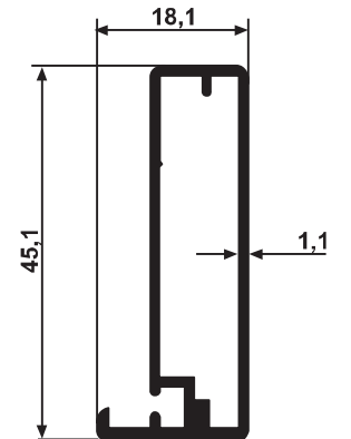
YG 2340 0,413 kg/m
