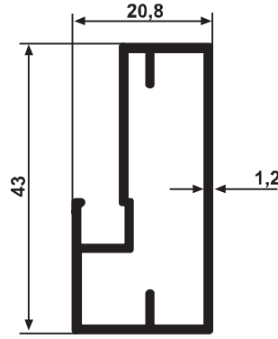
YG 3092 0,461 kg/m
