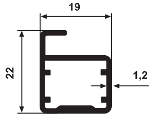
YG 2369 0,272 kg/m
