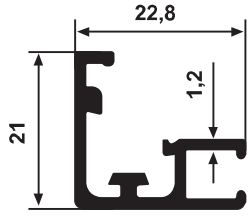
YG 2200 0,291 kg/m
