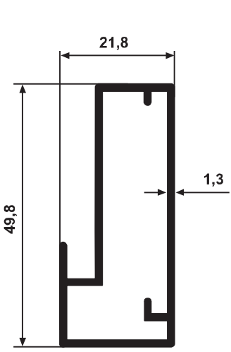
YG 1926 0,541 kg/m
