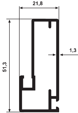
YG 2117 0,581 kg/m
