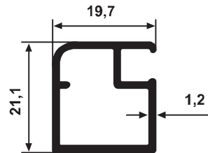
YG 3983 0,275 kg/m
