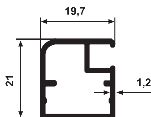
YG 3091 0,291 kg/m
