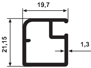
YG 2923 0,301 kg/m
