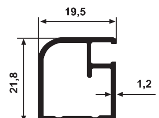
YG 4127 0,278 kg/m
