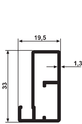
YG 2621 0,369 kg/m
