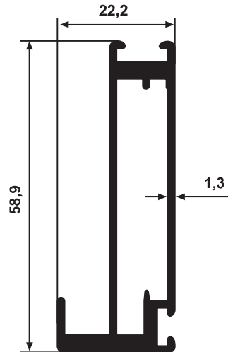
YG 2897 0,744 kg/m
