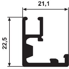
YG 1784 0,140 kg/m
