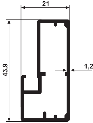
YG 2010 0,470 kg/m
