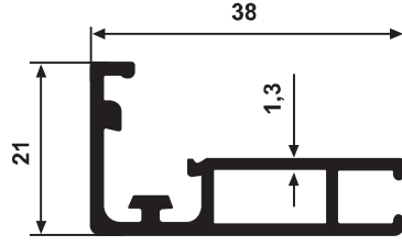
YG 2201 0,415 kg/m
