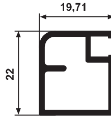
YG 2112 0,312 kg/m
