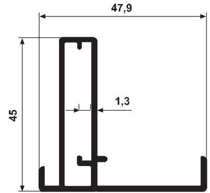
YG 2193 0,586 kg/m
