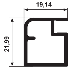
YG 1556 0,297 kg/m
