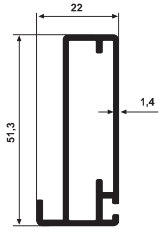
YG 3944 0,587 kg/m
