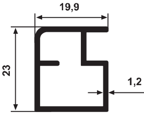
YG 2636 0,296 kg/m
