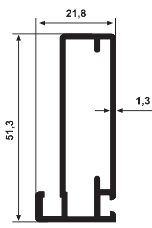
YG 2113 0,556 kg/m
