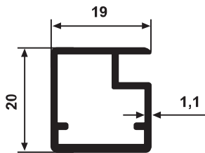
YG 2706 0,262 kg/m
