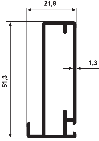
YG 1591 0,538 kg/m
