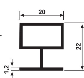
YG 1963 0,285 kg/m
