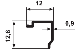
YG 2183 0,063 kg/m
