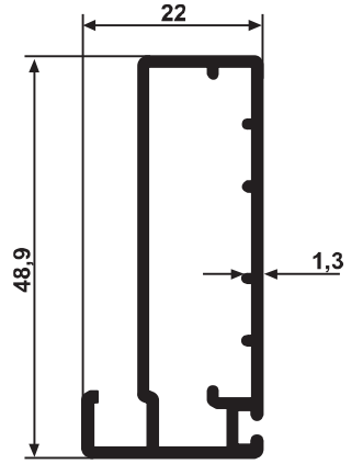
YG 2103 0,510 kg/m
