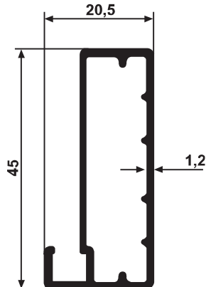
YG 2115 0,419 kg/m
