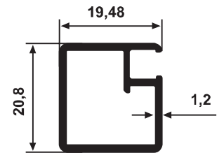
YG 4127 0,278 kg/m
