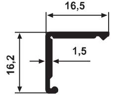
YG 2145 0,121 kg/m
