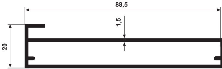
YG 3985 0,897 kg/m
