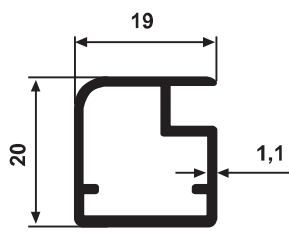
YG 3421 0,258 kg/m
