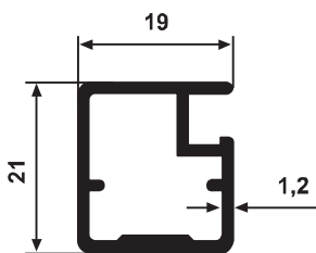
YG 2736 0,314 kg/m
