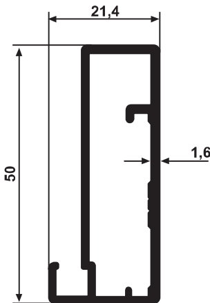
YG 1596 0,586 kg/m
