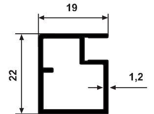
YG 2520 0,280 kg/m
