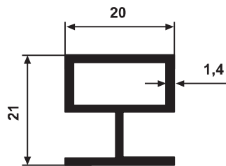
YG 2091 0,323 kg/m
