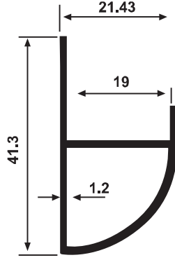
YG 4334 0,336 kg/m
