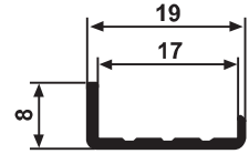
YG 2613 0,085 kg/m
