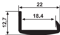
YG 2308 0,187 kg/m
