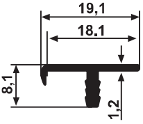
YG 2680 0,111 kg/m
