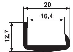
YG 2366 0,174 kg/m
