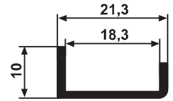
YG 2227 0,131 kg/m
