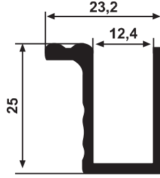
YG 1569 0,337 kg/m
