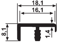
YG 2128 0,133 kg/m
