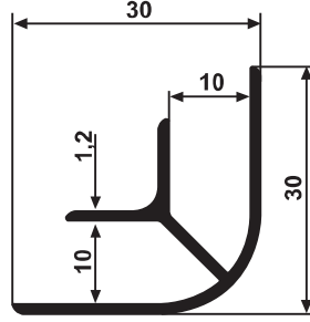
YG 2925 0,287 kg/m
