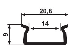
YG 2902 0,108 kg/m
