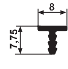
YG 4298 0,060 kg/m
