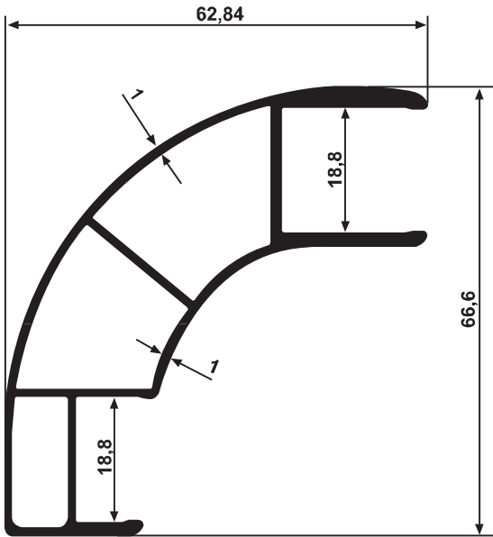
YG 3267 0,897 kg/m
