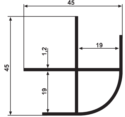
YG 4172 0,487 kg/m
