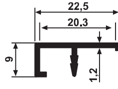
YG 3981 0,136 kg/m
