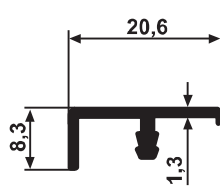
YG 2433 0,133 kg/m
