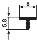
YG 3073 0,046 kg/m
