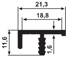
YG 1512 0,189 kg/m
