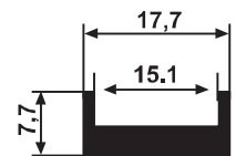
YG 2102 0,197 kg/m
