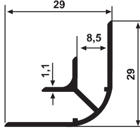
YG 2874 0,237 kg/m
