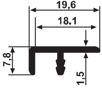
YG 2278 0,133 kg/m
