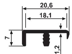
YG 2683 0,132 kg/m
