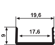
YG 2412 0,096 kg/m
