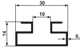
YG 3015 0,210 kg/m
