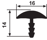
YG 2081 0,179 kg/m
