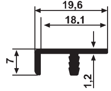
YG 2682 0,124 kg/m
