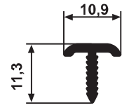
YG 2018 0,088 kg/m
