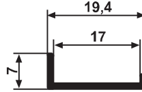
YG 3342 0,087 kg/m
