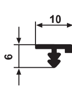
YG 3779 0,059 kg/m
