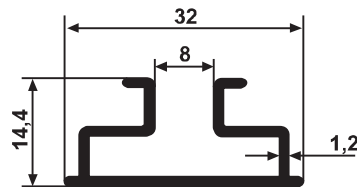
YG 3102 0,262 kg/m
