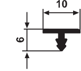
YG 2395 0,051 kg/m
