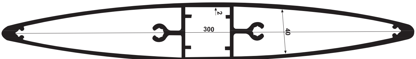
YS 6780 4,170 kg/m Ölçek 4/5
